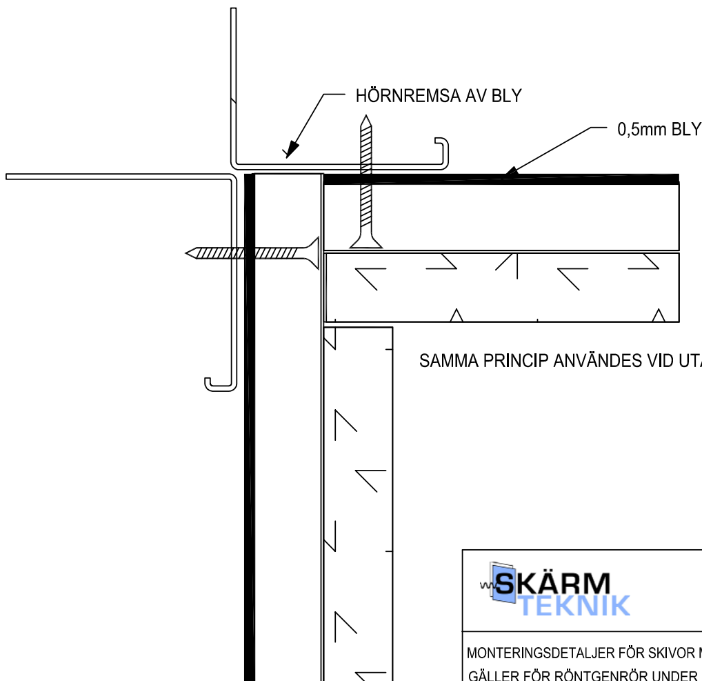
HORISONTALSEKTION
